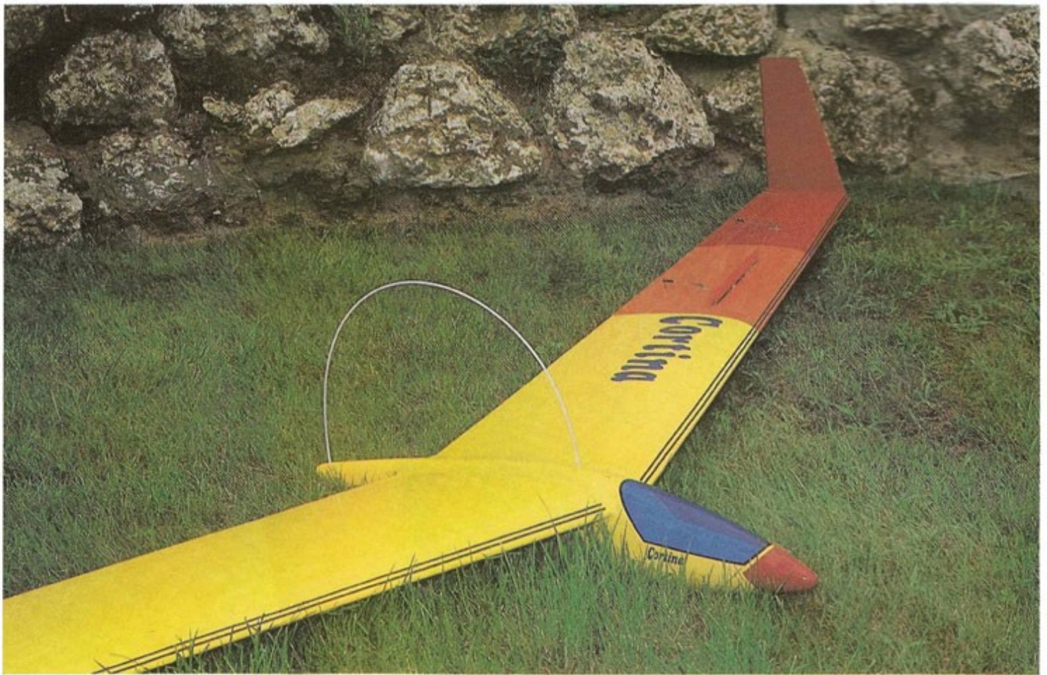
Notez ci-dessus le tube replié au-dessus du fuselage qui permet de loger l'antenne bien déployée. Ci-dessous le fuselage ne renferme en fait que deux servos : celui des aérofreins que l'on voit ici et celui du crochet de remorquage. Les servos d'ailerons et de profondeur sont logés dans les ailes et raccordés au récepteur via des rallonges dont une partie bobinée autour d'un tore en ferrite pour éviter tout parasite.
