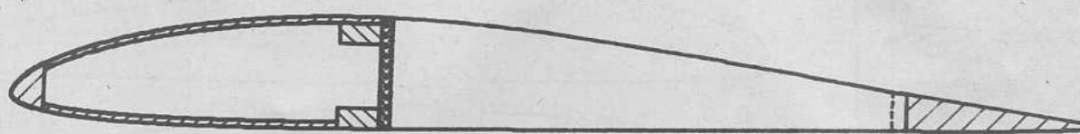
COUPE BB
