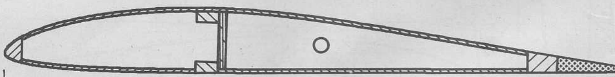
COUPE AA
