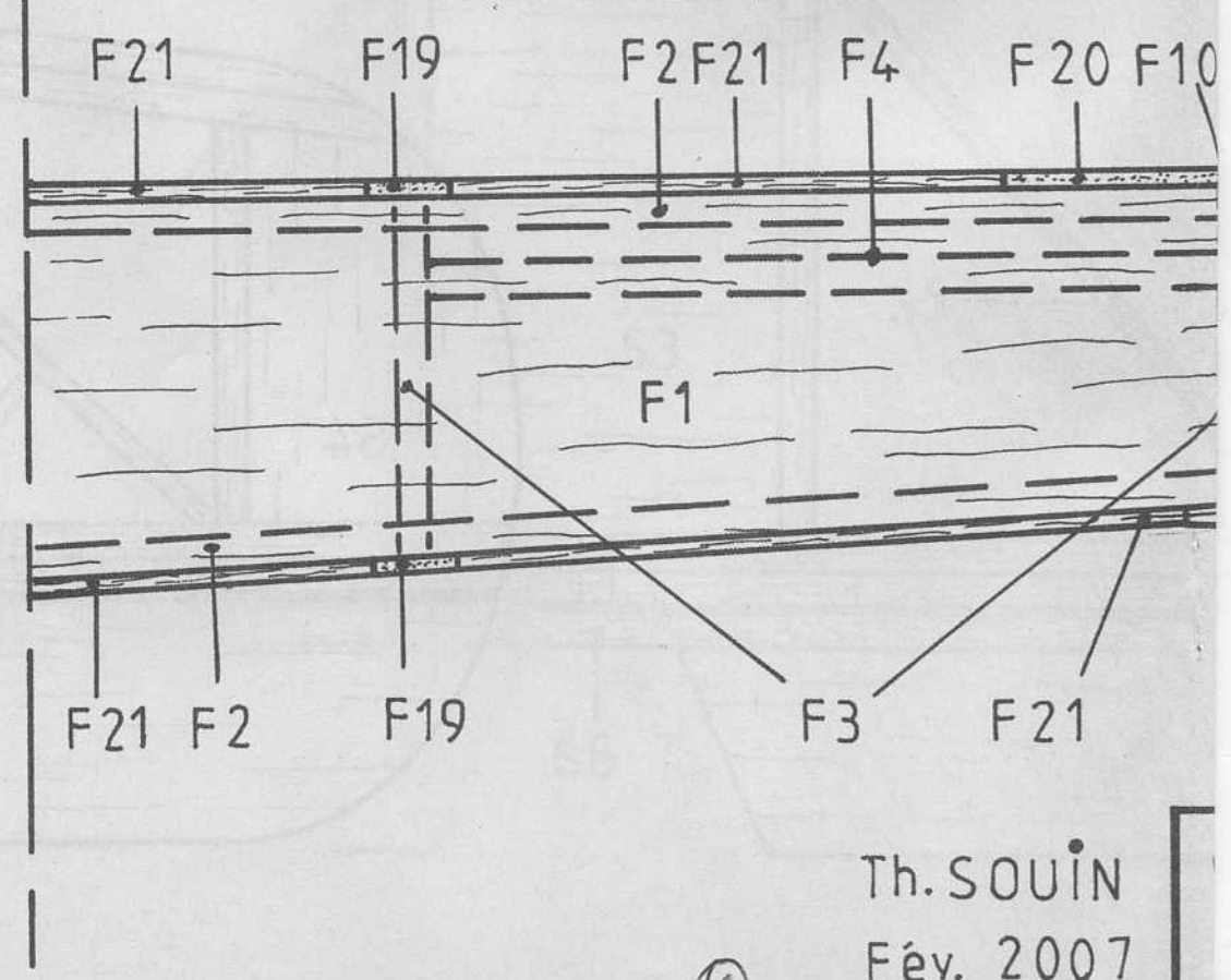
Coupe D-D.
