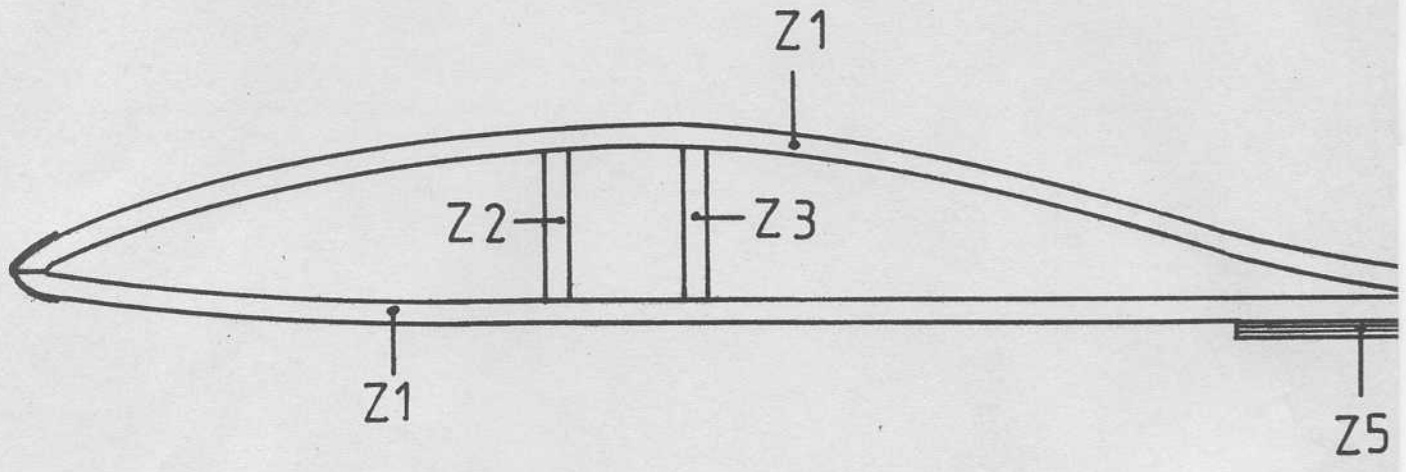
Coupe A-A (propulsion installée).
